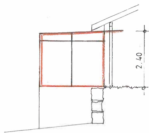
SÜD
